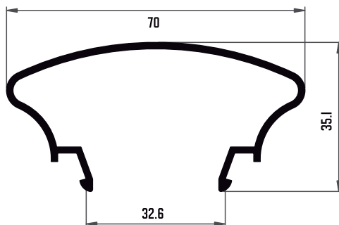
10022 PASAMANOS 70 MM
