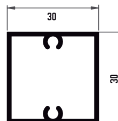
10021 BARANDILLA 30X30 MM
